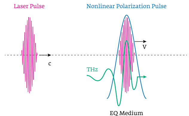
Рис. 3. Оптическое выпрямление Fig. 3. Optical rectification
