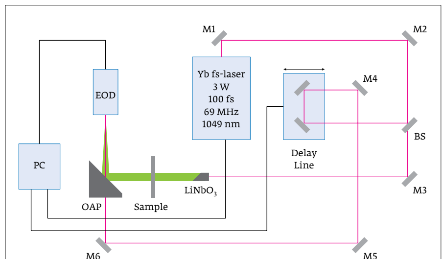
Рис. 2. Принципиальная оптическая схема ИТС-1 Fig. 2. General optical layout of the PTS-1
