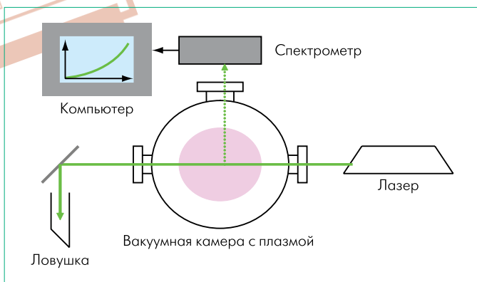
Рис. 1 Схема установки томсоновского рассеяния для измерения температуры электронов в плазме
