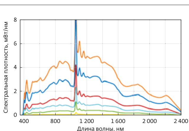
Рис.1. Суперконтинуумные источники, работающие с различной частотой повторения импульсов, обеспечивают высокую повторяемость формы спектра. При этом средняя мощность излучения пропорциональна спектральной плотности
